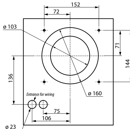
Розмітка отворів під кріплення виробу
