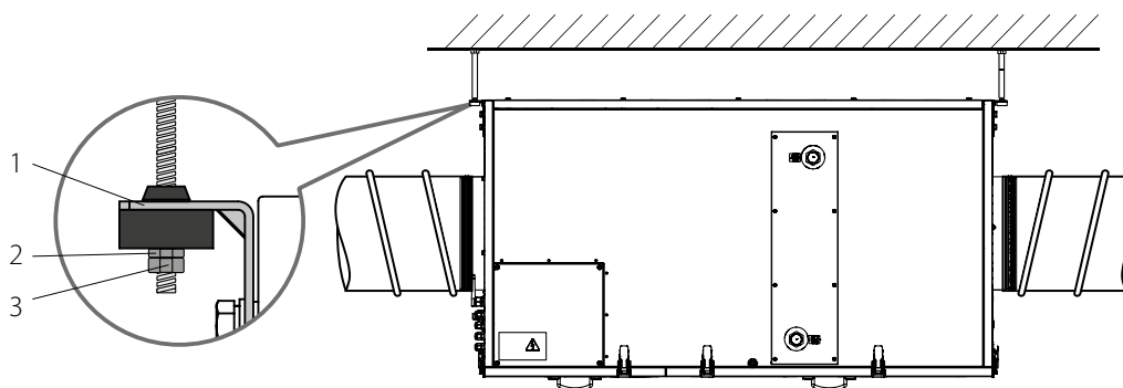
1 — монтажний кронштейн; 2 — гайка; 3 — контргайка
