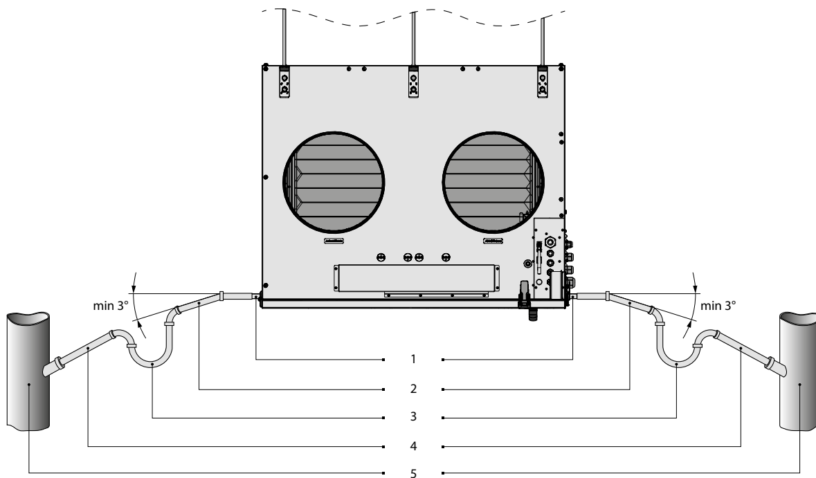
1 – Трубка для відведення конденсату; 2 – Труба; 3 – Сифон; 4 – Труба; 5 – Каналізація
